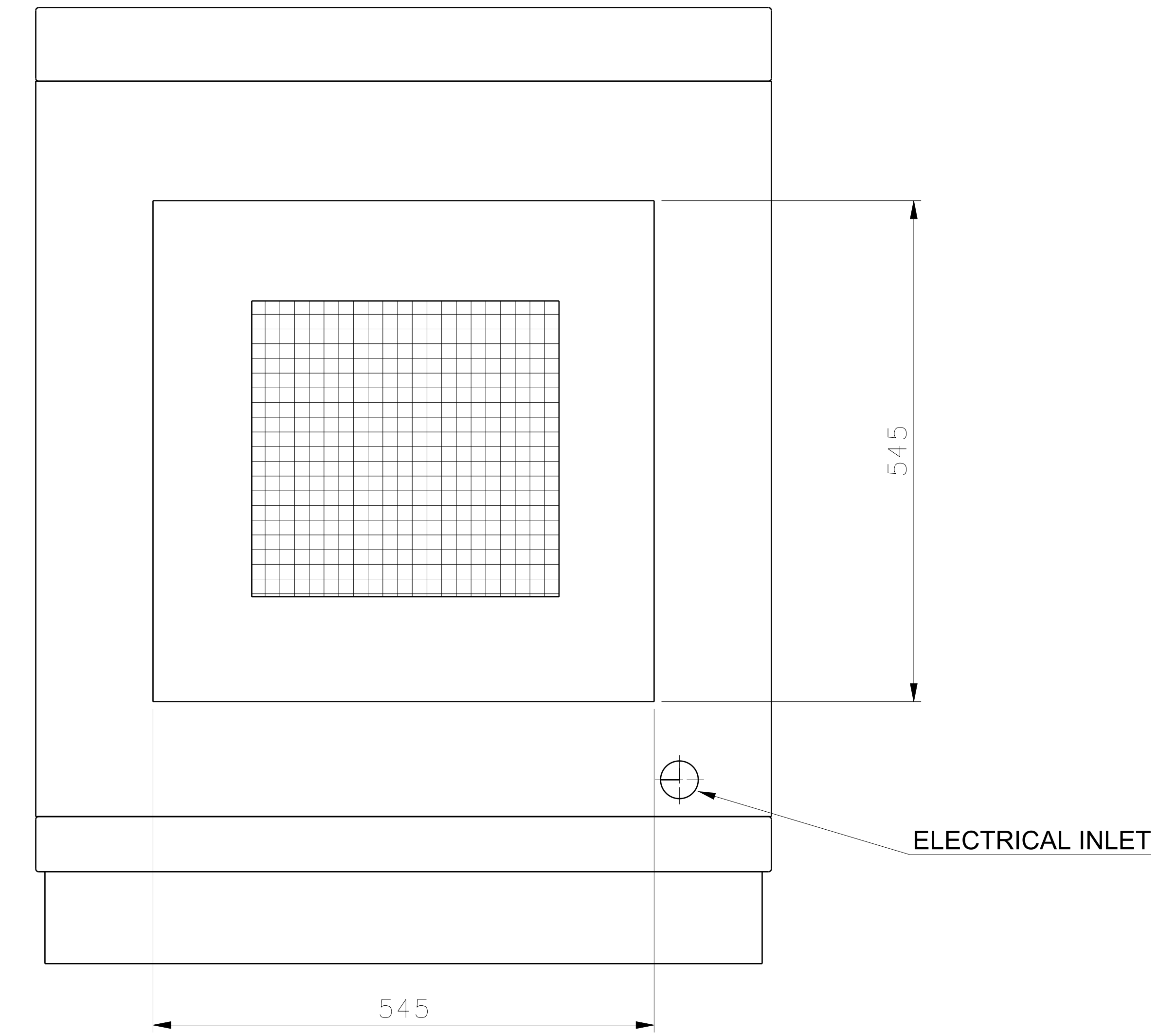
Left view Scale: 1:4
