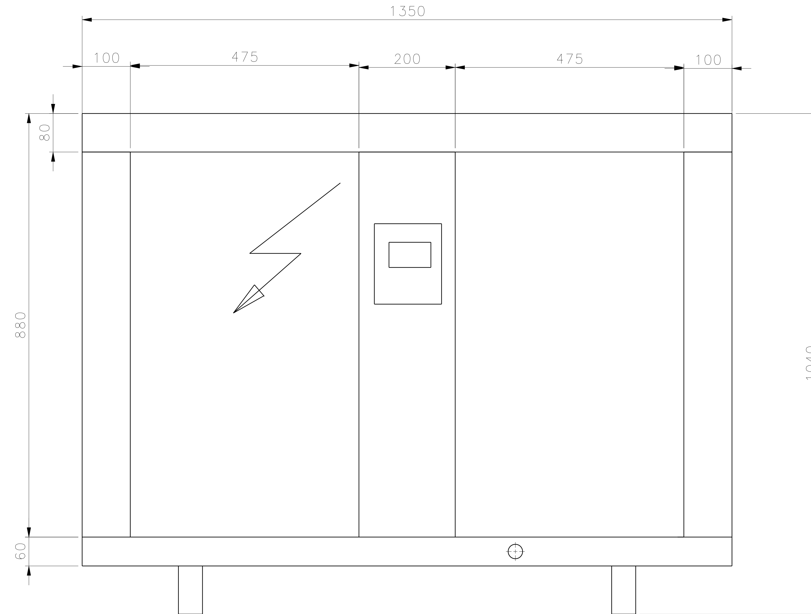
Front view Scale: 1:4
