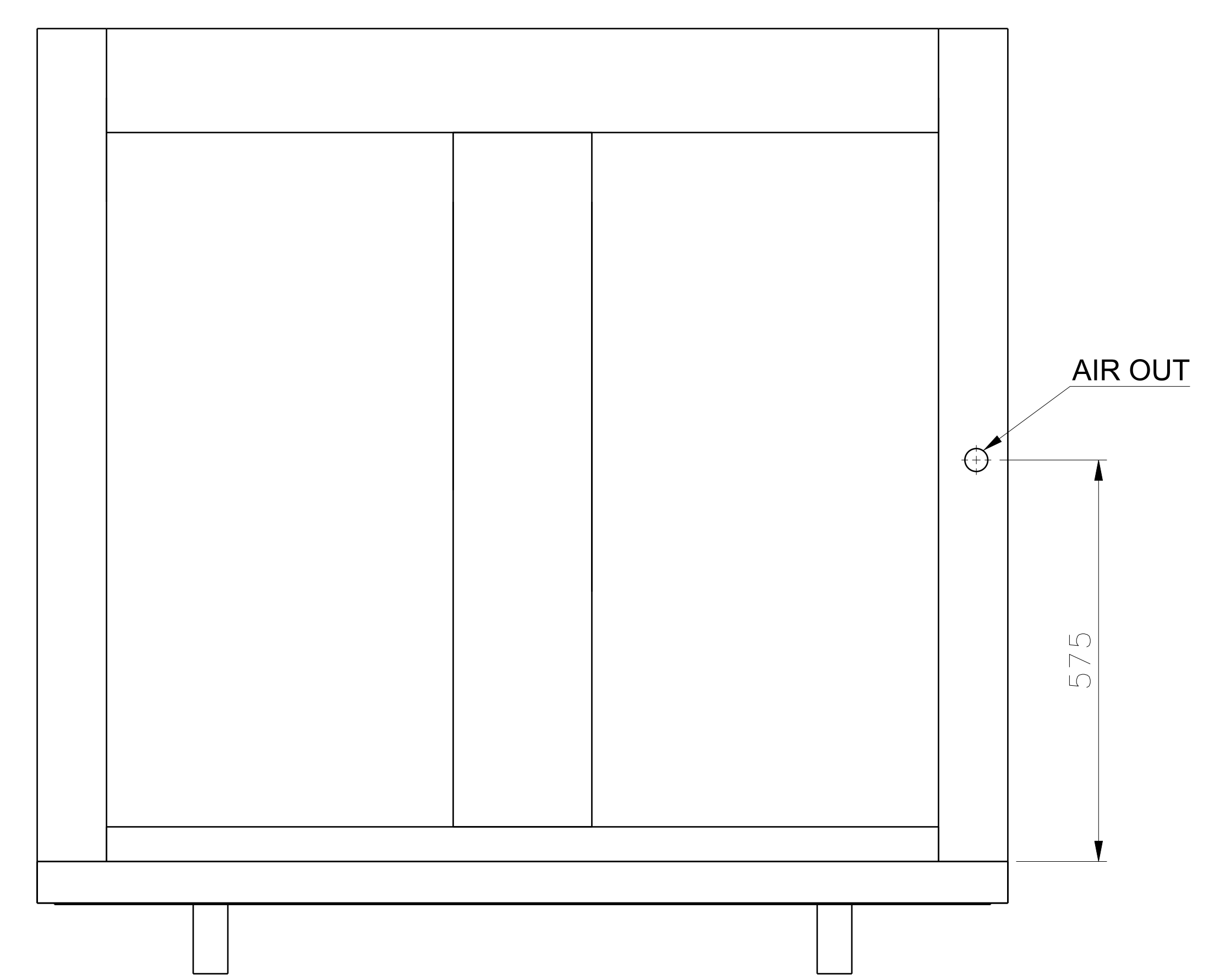
Rear view[2] Scale: 1:6
