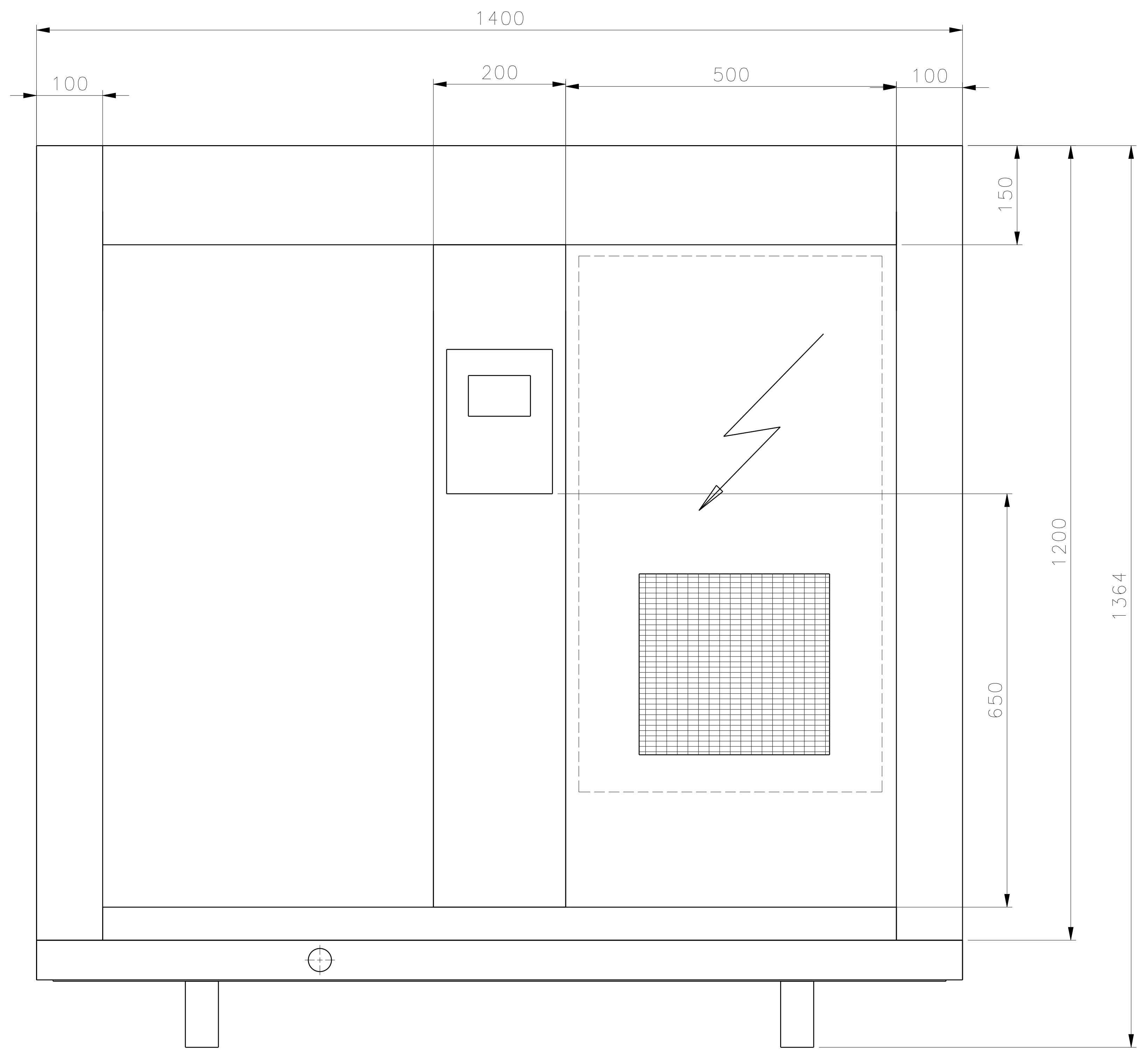
Front view Scale: 1:4
