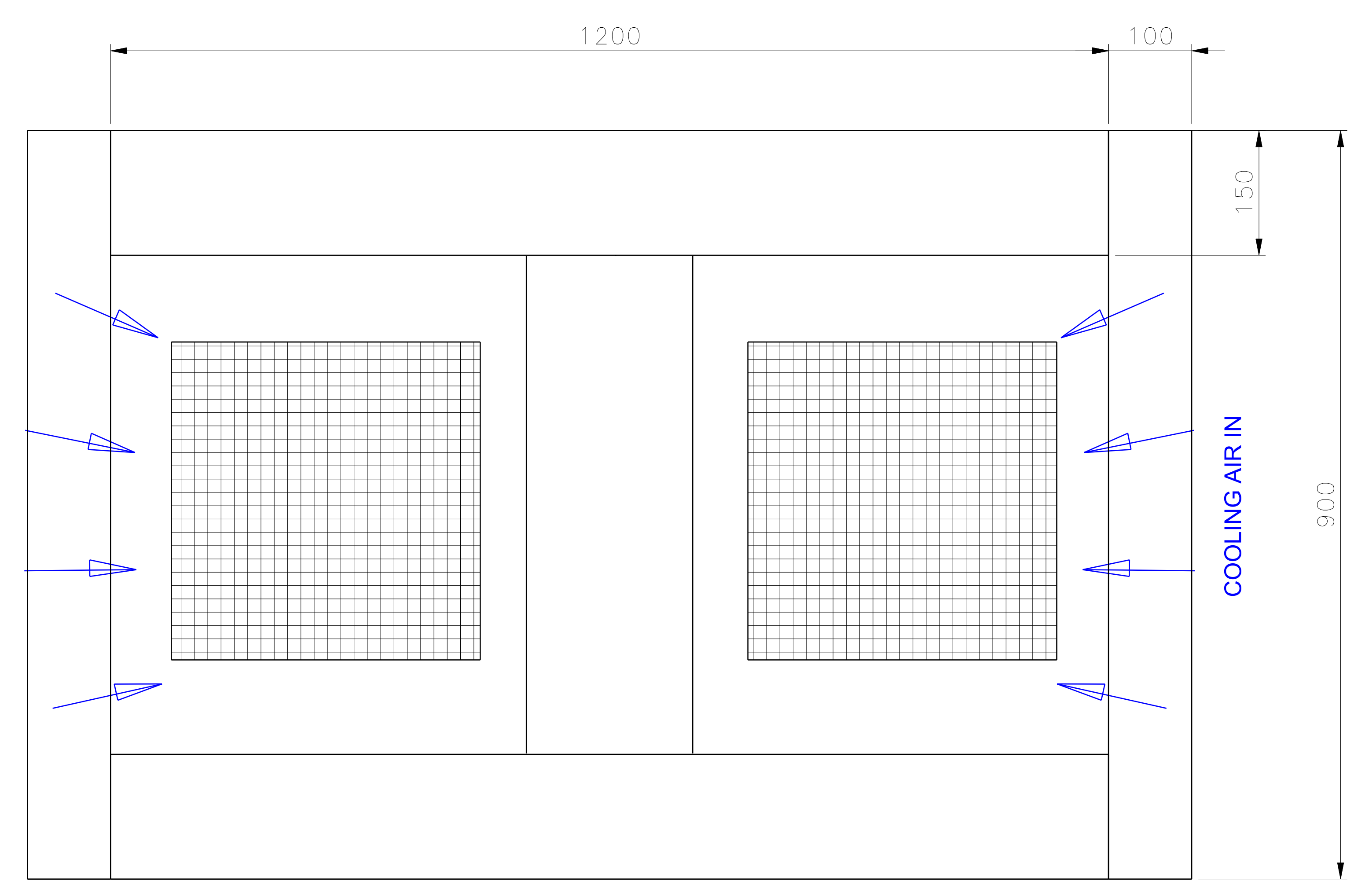
Top view Scale: 1:4
