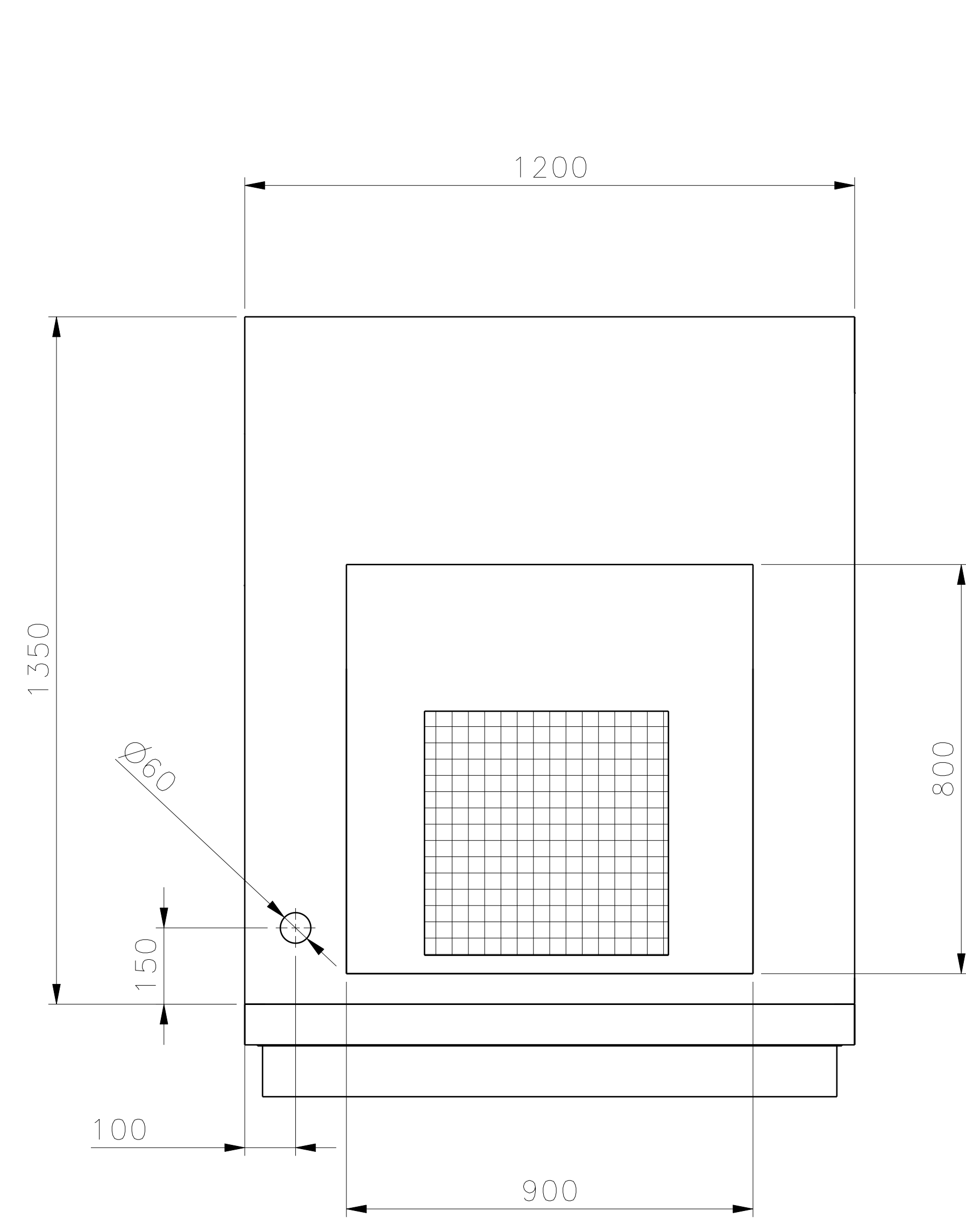
Right view Scale: 1:8
