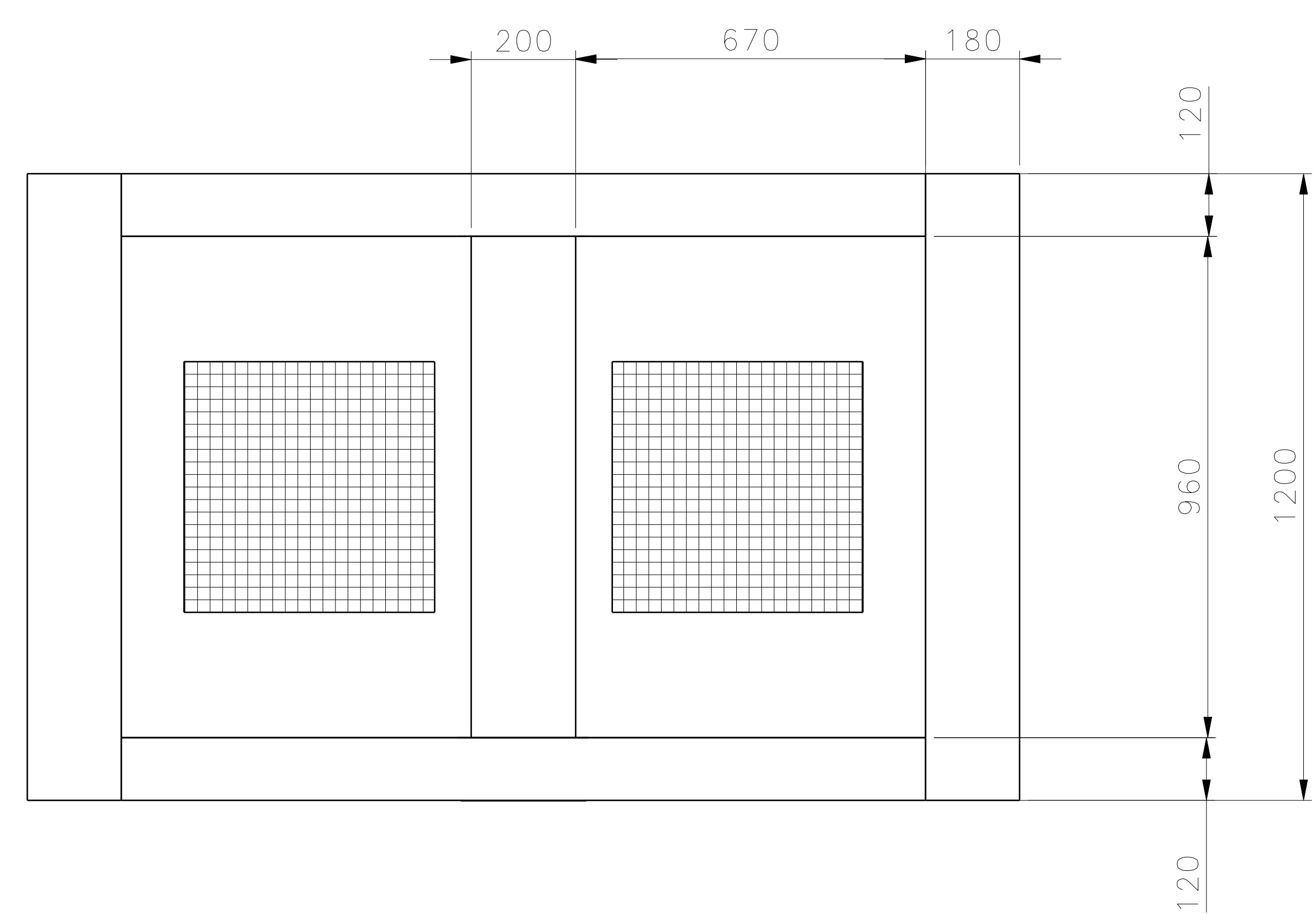
Top view[2] Scale: 1:8
