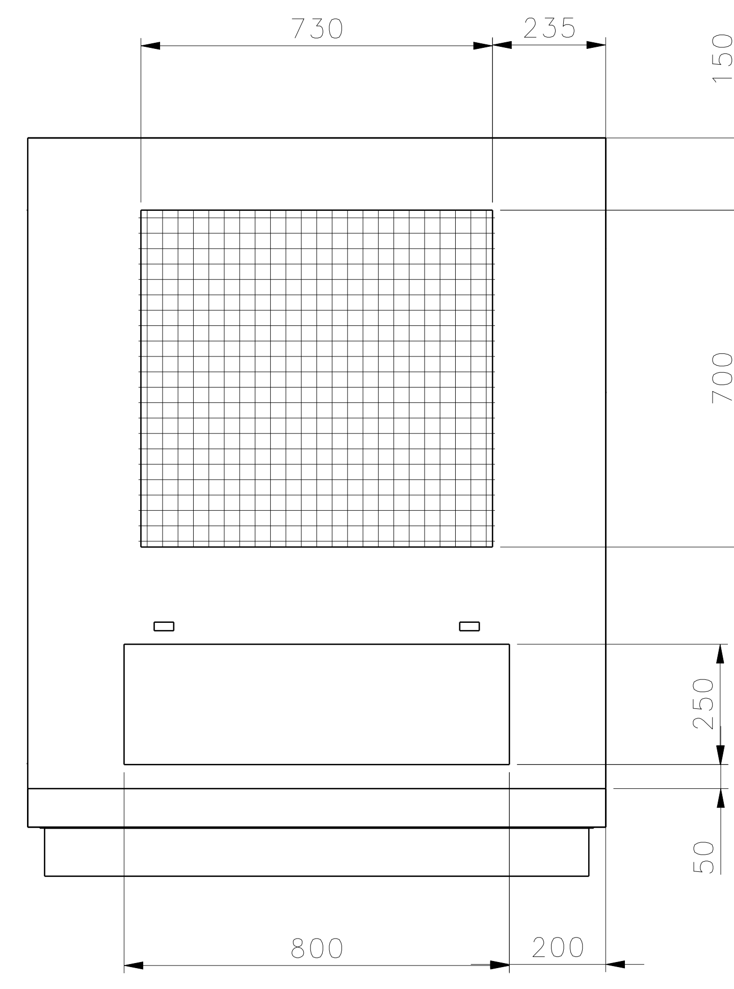
Left view Scale: 1:8
