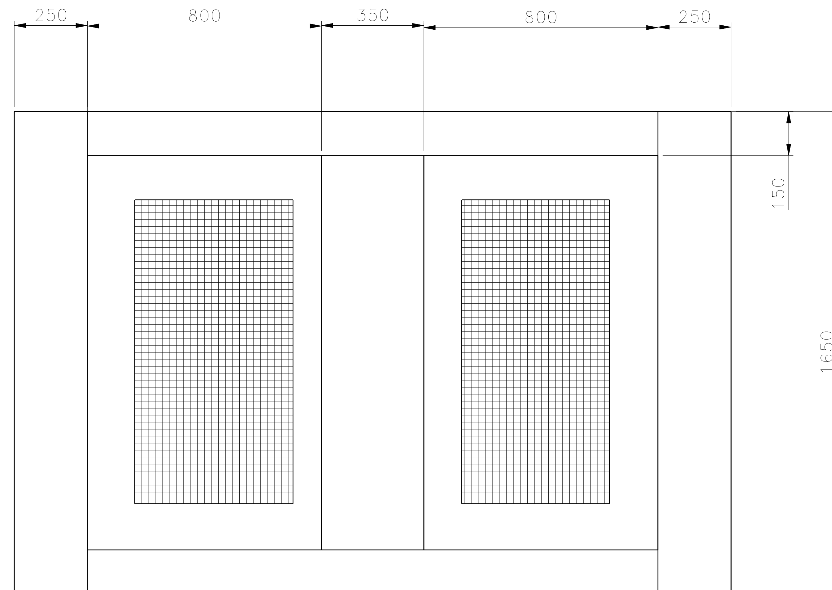
Top view Scale: 1:8
