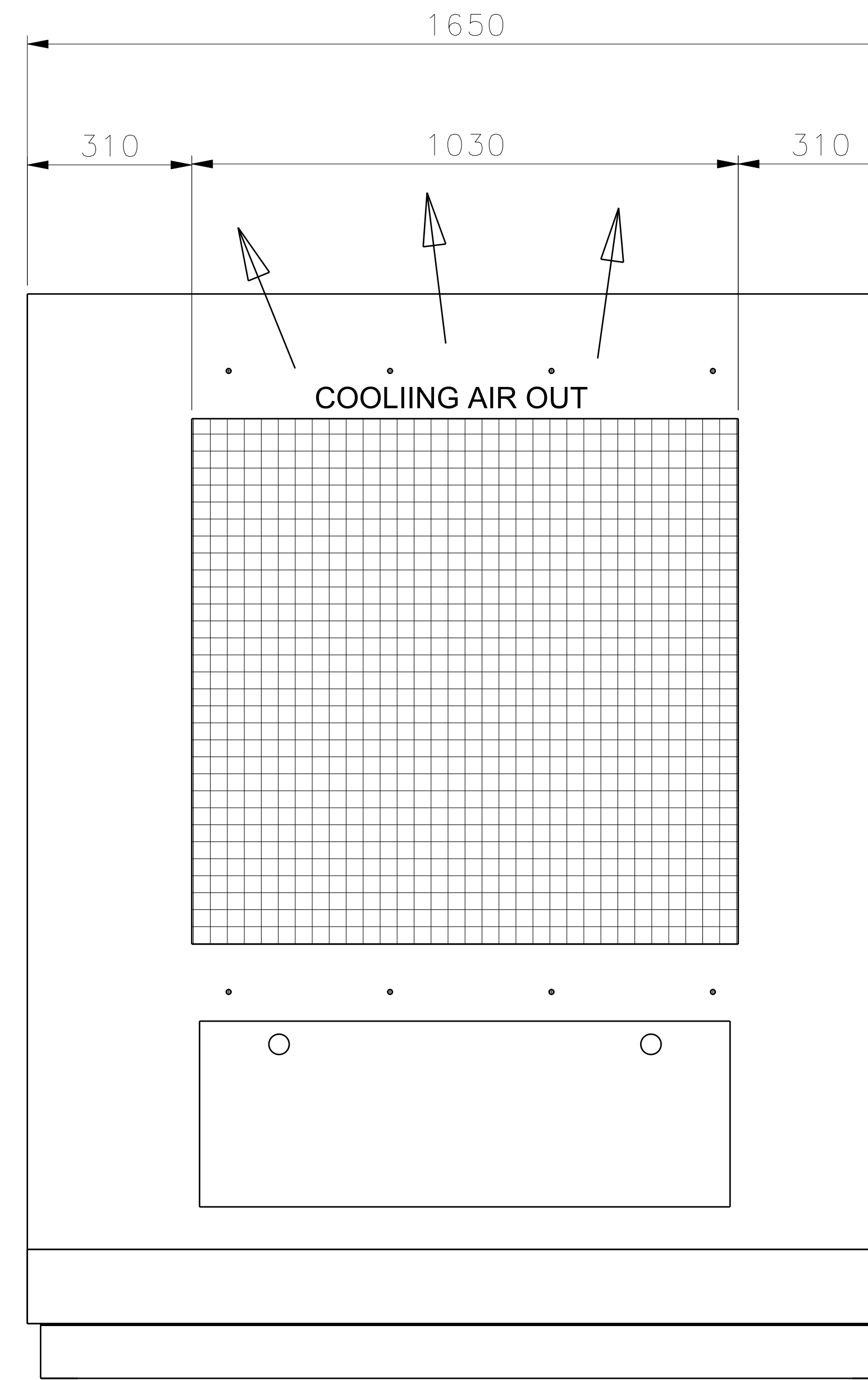
Left view Scale: 1:8
