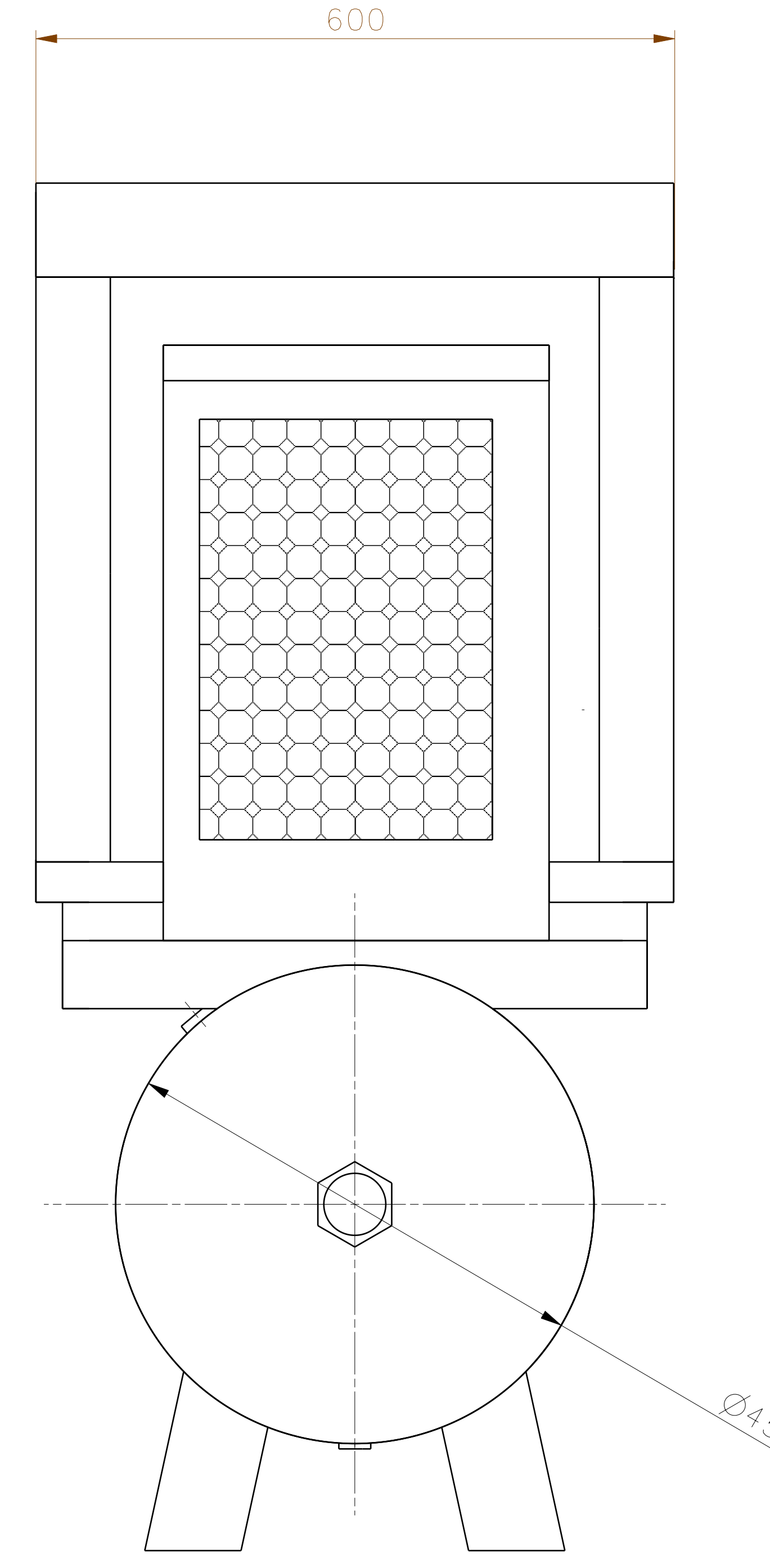
Left view Scale: 1:4
