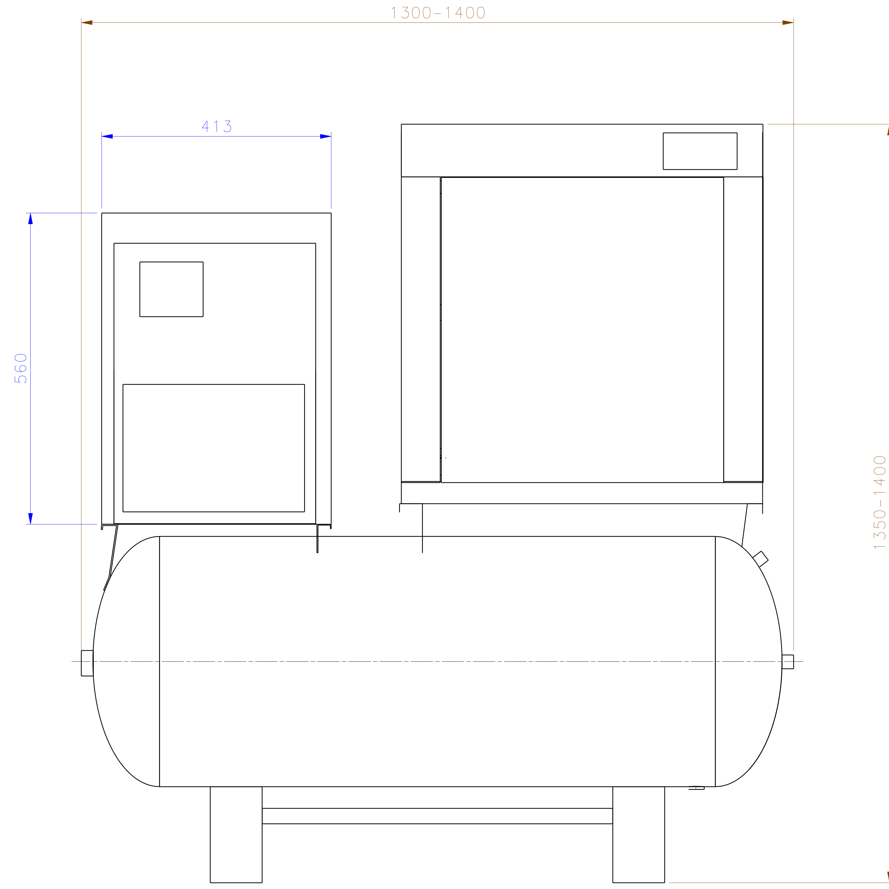
Front view Scale: 1:4
