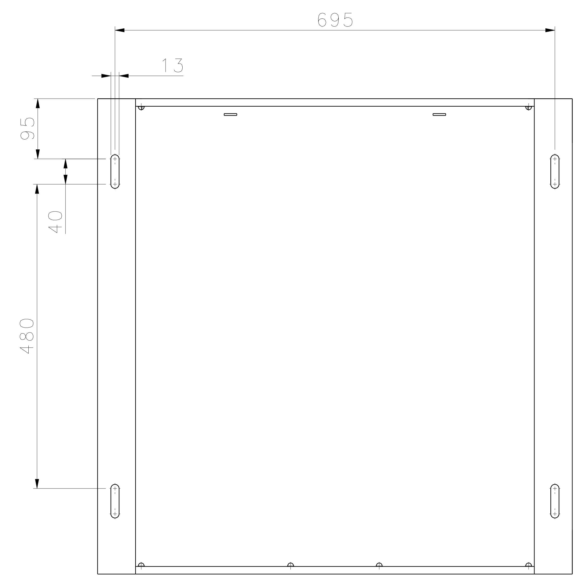
Bottom view Scale: 1:3
