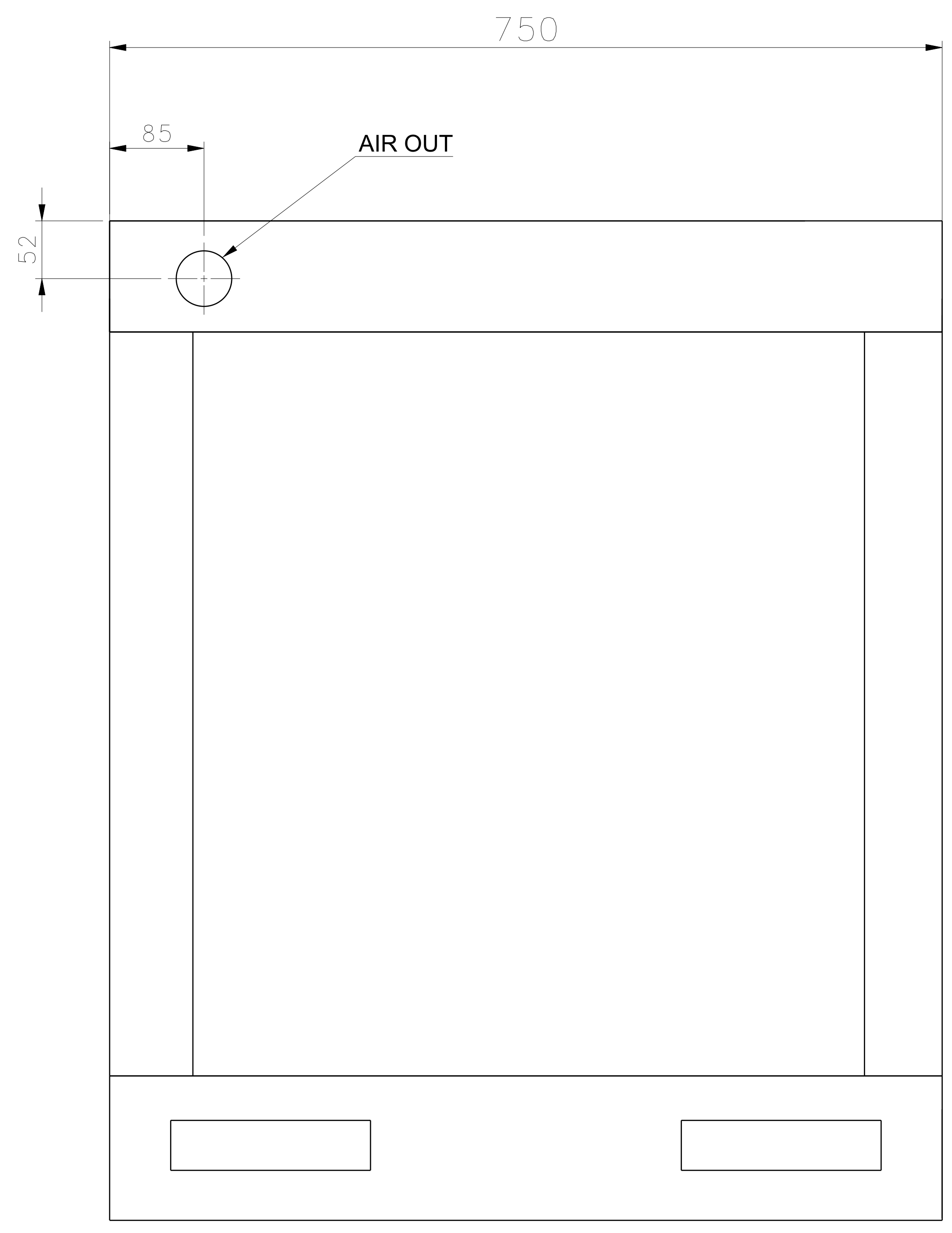
Left view Scale: 1:3
