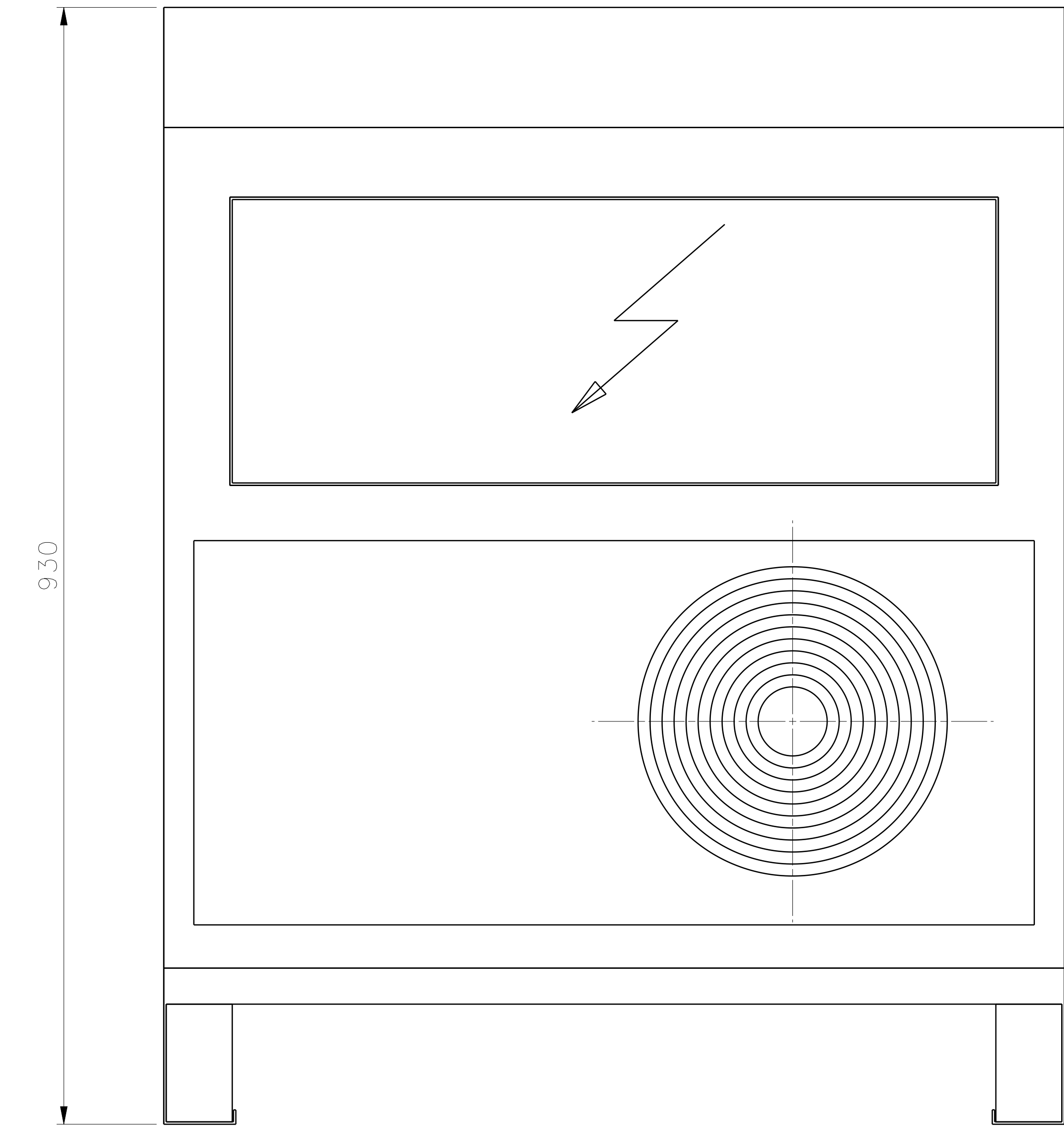
Rear view Scale: 1:3
